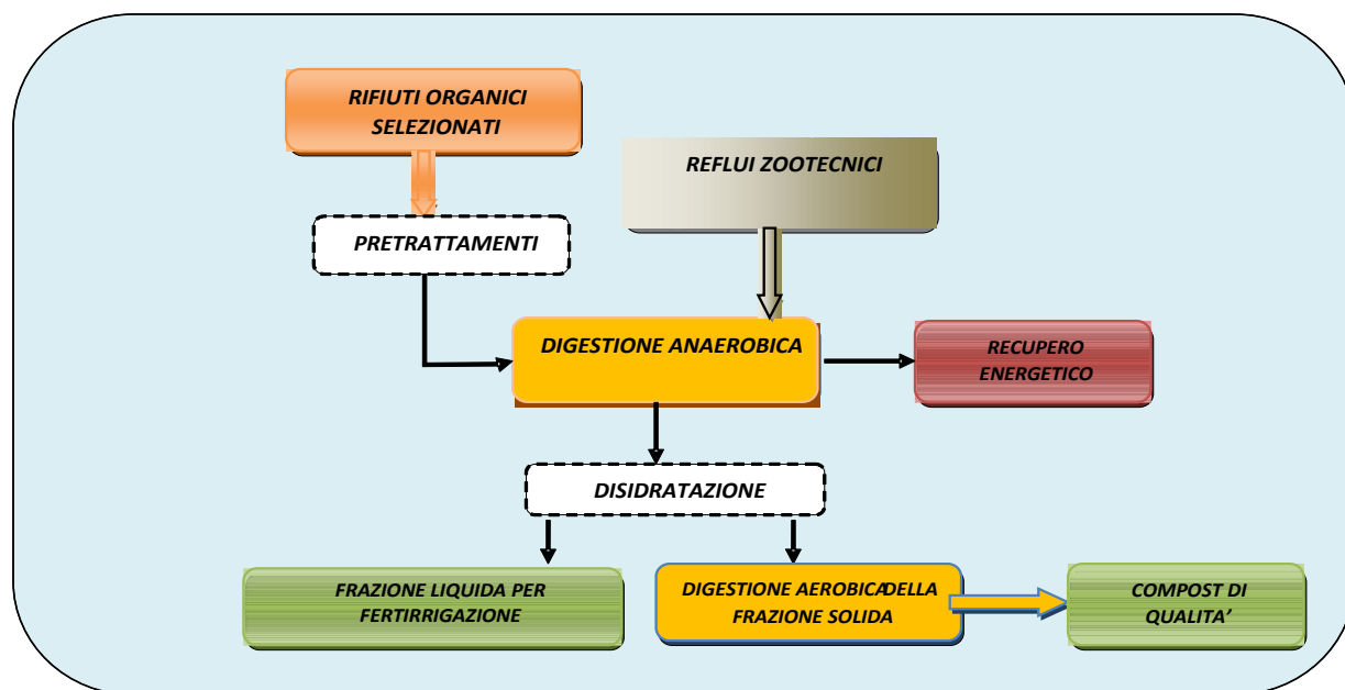
Schema generale di flusso per il recupero energetico da biomasse
