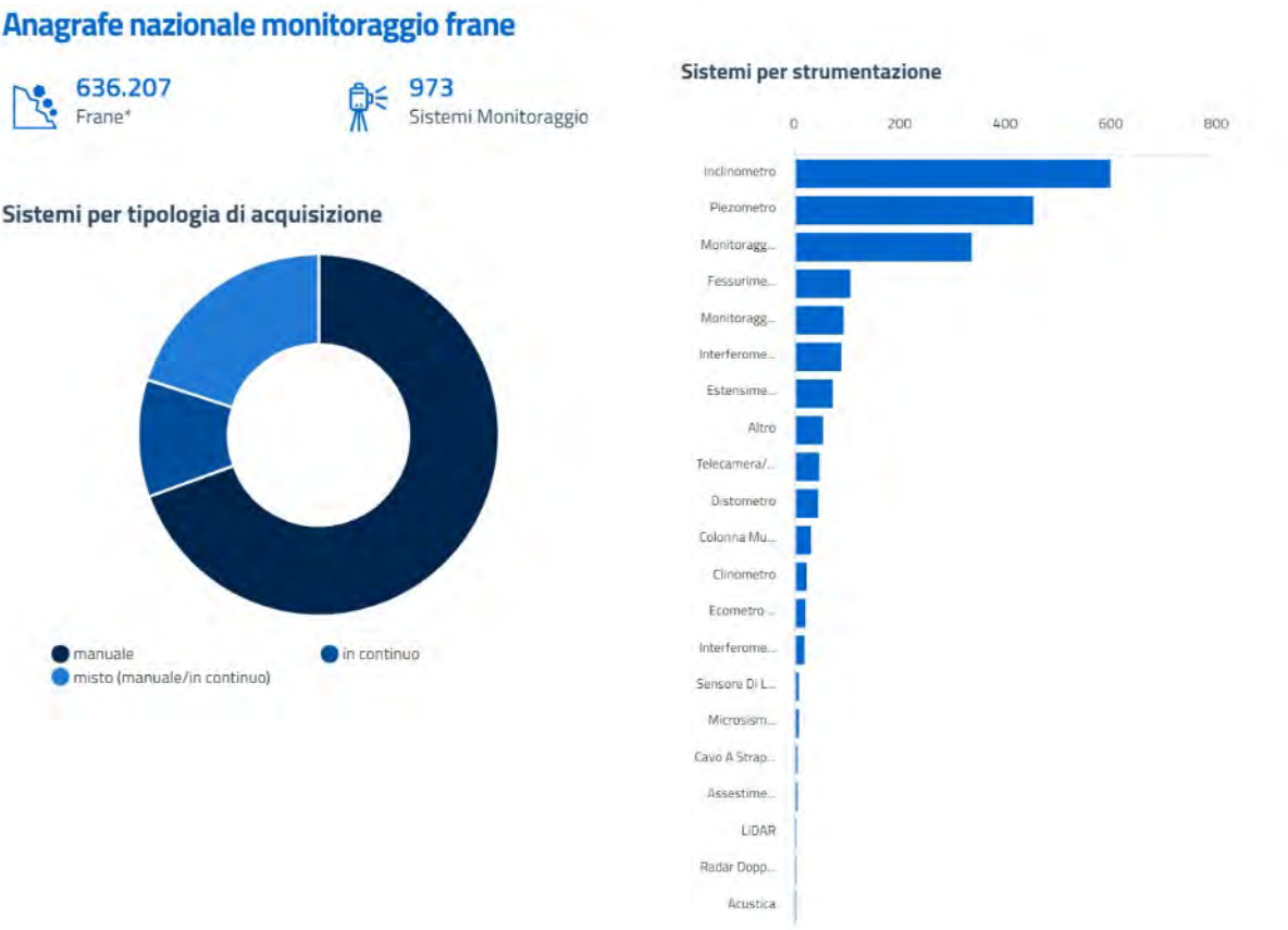
Figura 7.2 – Anagrafe nazionale dei sistemi di monitoraggio in situ delle frane: distribuzione percentuale della tipologia di acquisizione dati dei sistemi di monitoraggio; tipologia di strumentazione utilizzata nei sistemi di monitoraggio
